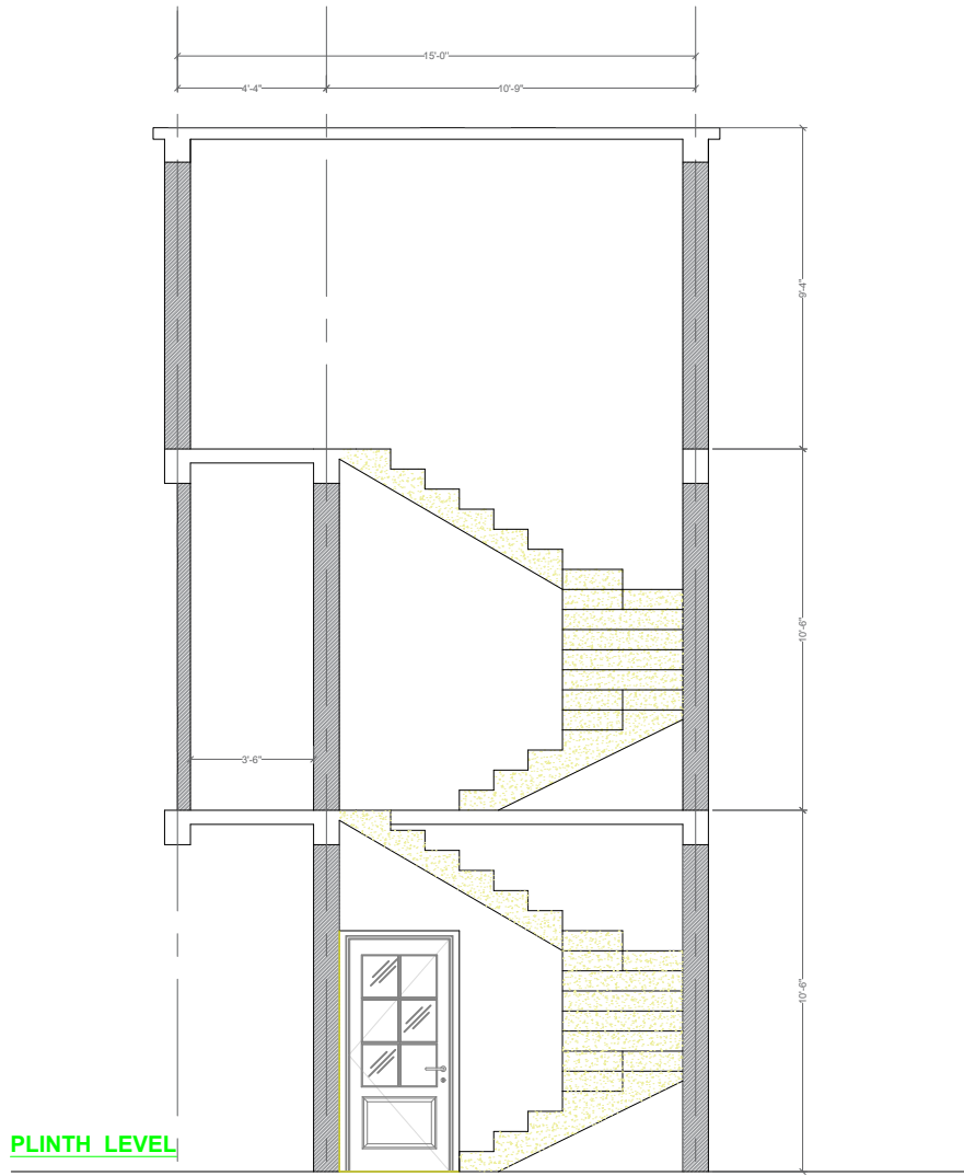
SECTION A-A
