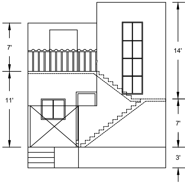
ELEVATION
